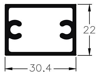
478 - Parante Angosto peso: 0,51 Kg/m
