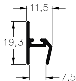
438 - Cierre vidrio 180° peso: 0,15 Kg/m
