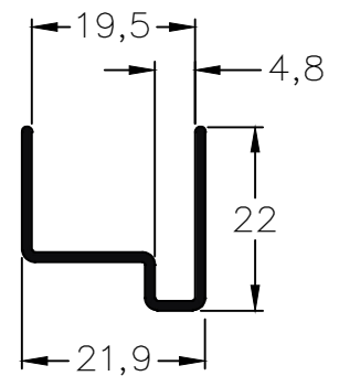
158 - Cantenera p/18 mm peso: 0,20 Kg/m
