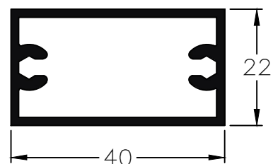
476 - Parante peso: 0,61 Kg/m
