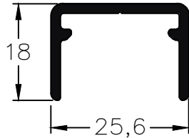
401 - Remate vidrio 10+10 Peso: 0,29 Kg/m
