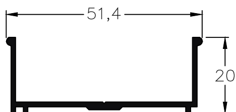
943 - Jamba de Mampara peso: 0,32 Kg/m
