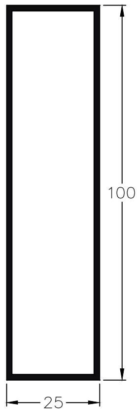
461 - Tubo 100 x 25 mm e: 1,5 peso: 0,99 Kg/m
