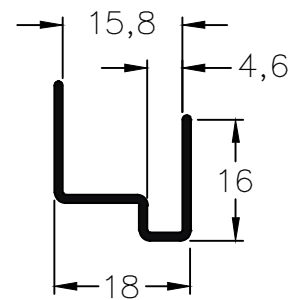
156 - Cantenera p/15mm peso: 0,16 Kg/m
