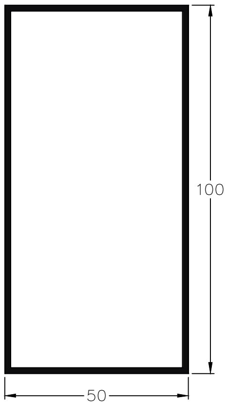
454 - Tubo 100 x 50 mm e: 1,6 peso: 1,27 Kg/m
