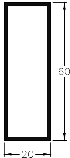
812 - Tubo 60 x 20 mm peso: 0,63 Kg/m
