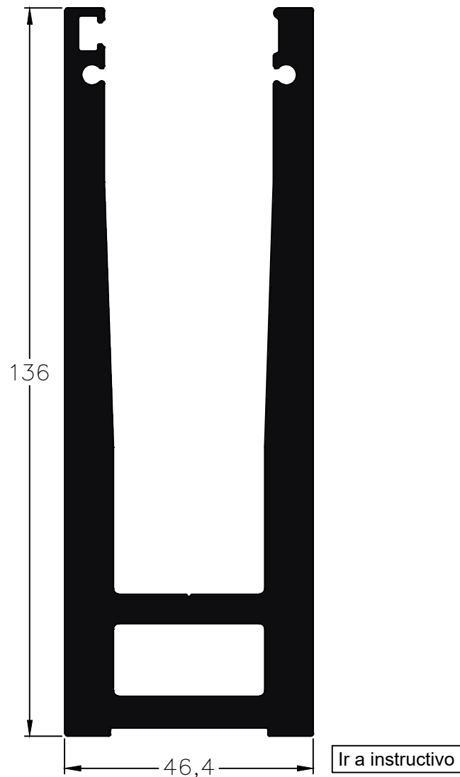
423 - Base Baranda SPU Largo Std.: 3000 mm Peso: 6,88 Kg/m
