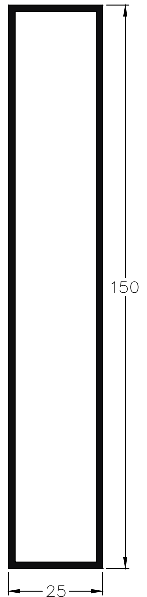
472 - Tubo 150 x 25 mm e: 1,7 peso: 1,58 Kg/m
