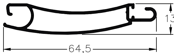
625 - Tablilla Cortina Común
