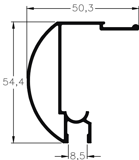
434 - Cabezal mampara corrediza peso: 0,62 Kg/m
