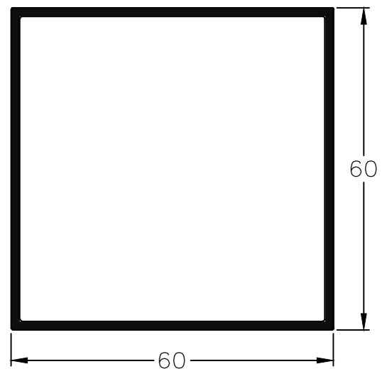
459 - Tubo 60 x 60 mm peso: 1,01 Kg/m
