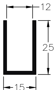
650 - U de 15 x 25 mm peso: 0,25 Kg/m
