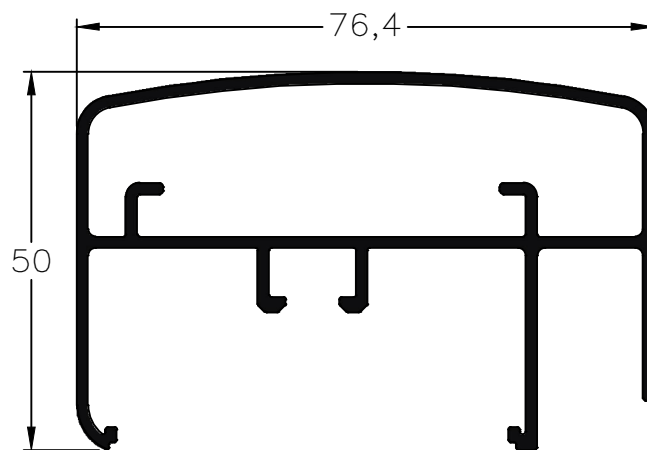
025 - Pasamanos Recto BBA peso: 1,24 Kg/m
