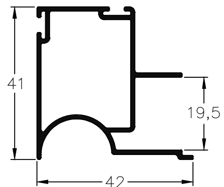
159 - Parante p/18mm Largo Std.: 5200 mm Peso: 0,54 Kg/m
